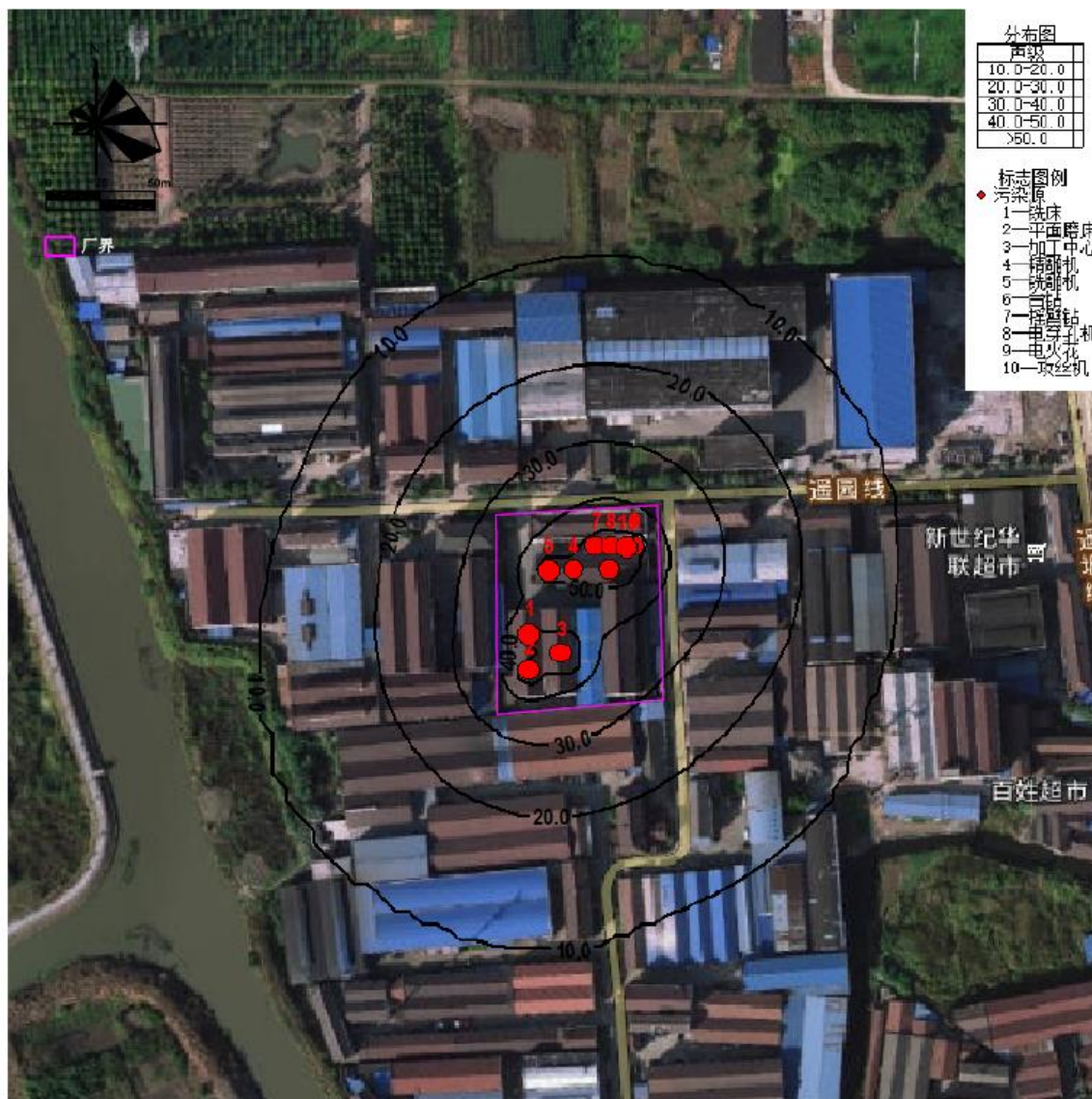
图 7-2 等声级线图
