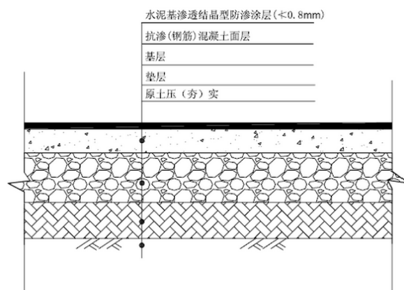
图 5-4 装置区地坪防渗结构示意图
