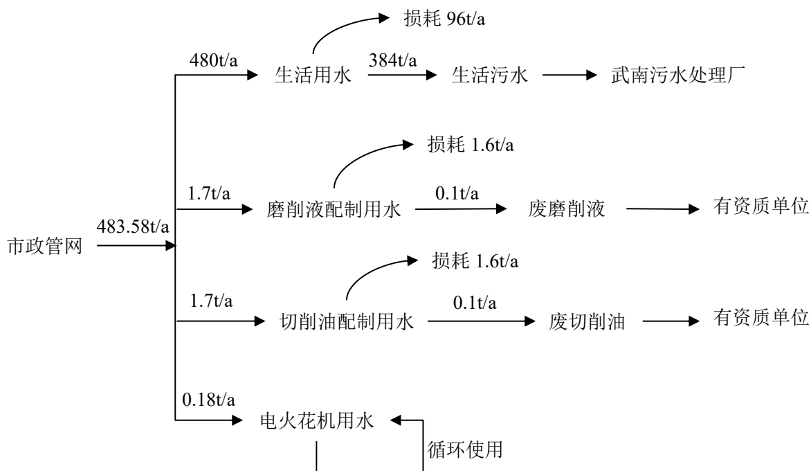
图 5-2 本项目水平衡图
