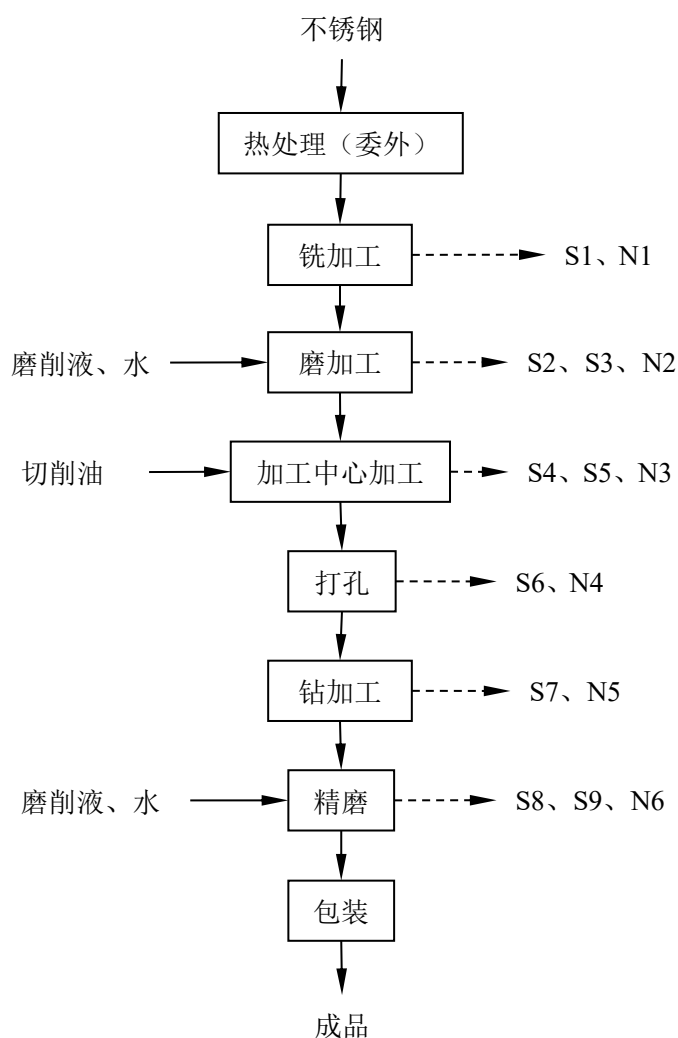
图 5-1 喷丝板和无纺机械配件生产工艺流程图
