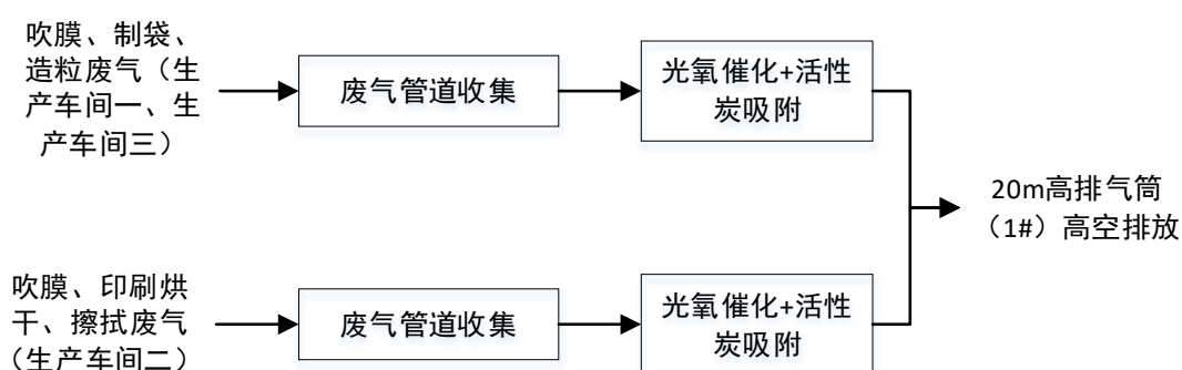
图 5-5 本项目废气处理工艺流程图
