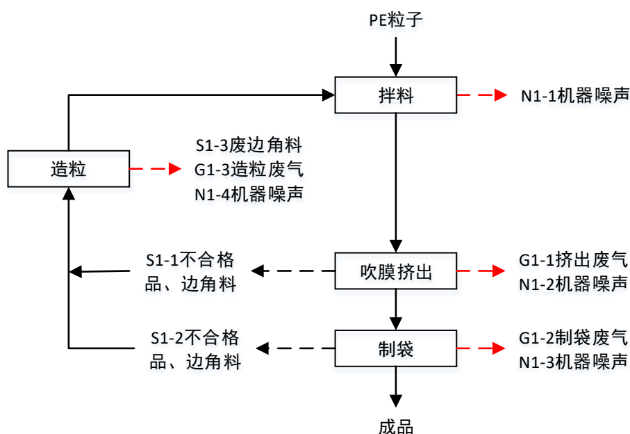
图 5-1 塑料包装袋生产工艺流程图
