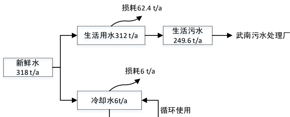
图 5-2 本项目水平衡图
