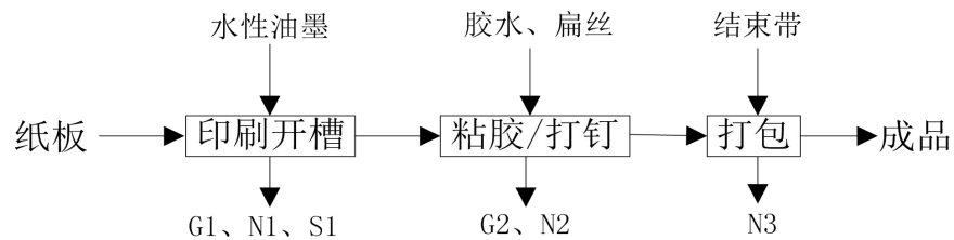
图2-2 纸箱生产工艺流程图
