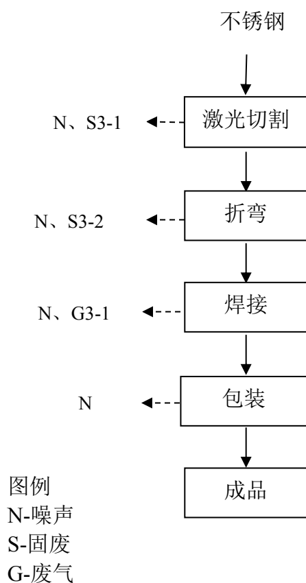
图 2-4 厨房用品、操作台加工工艺流程图
