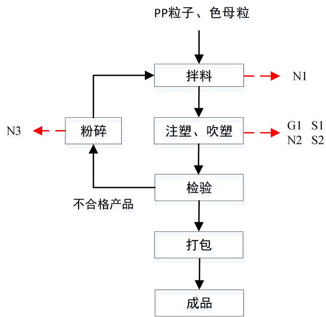
图 2-2 塑料桶生产工艺流程图
