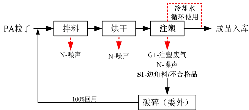
图2-1 塑料制品生产工艺流程图
