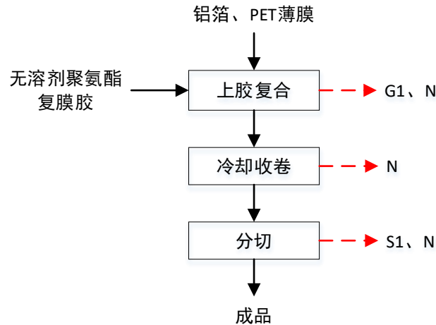
图 2 铝塑复合带生产工艺流程图 (注: Gn: 废气污染物; Sn: 固体废弃物; Nn: 噪声)
