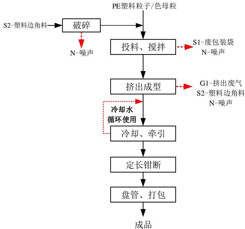
图 2-1 PE 管工艺流程图
