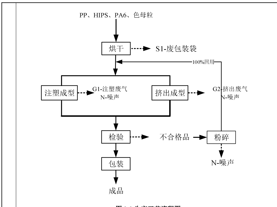
图 2-2 生产工艺流程图 (注: Gn: 废气污染物; Sn: 固体废弃物; Nn: 噪声)
