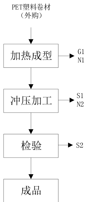
图 2-2 包装吸塑托盘生产工艺流程图
