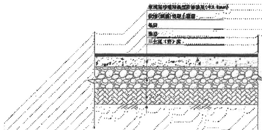
图 4-9 生产区地坪防渗结构示意图
