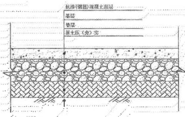
图 4-11 一般污染防治区典型防渗结构示意图
