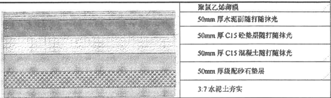
图 4-10 危废仓库防渗结构示意图
