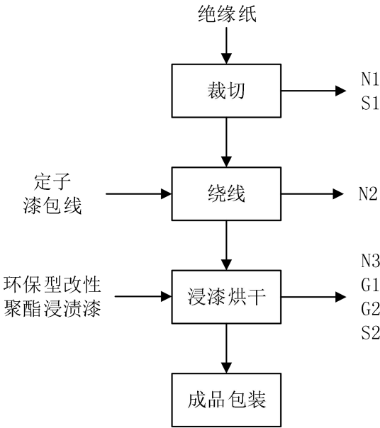
图 2-3 电机定子生产工艺流程图 (注：Gn：废气污染物；Sn：固体废弃物；N：噪声)
