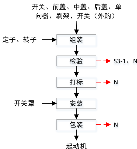
图 2-4 起动机总装生产工艺流程图 （注：Sn：固体废弃物；N：噪声）
