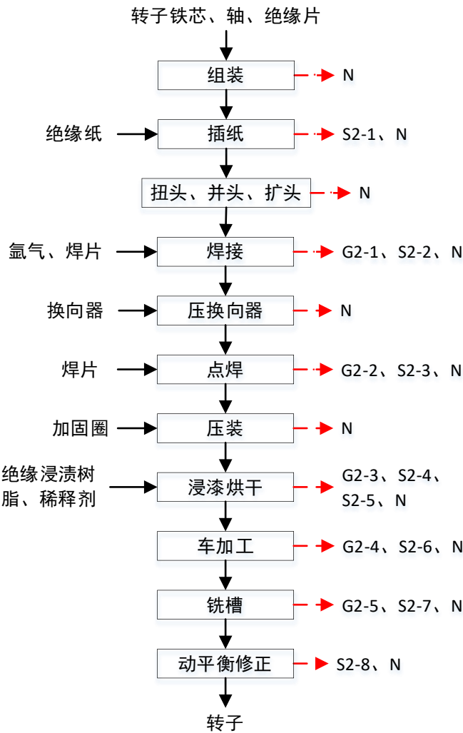
图 2-3 转子生产工艺流程图 （注：Gn：废气污染物；Sn：固体废弃物；N：噪声）
