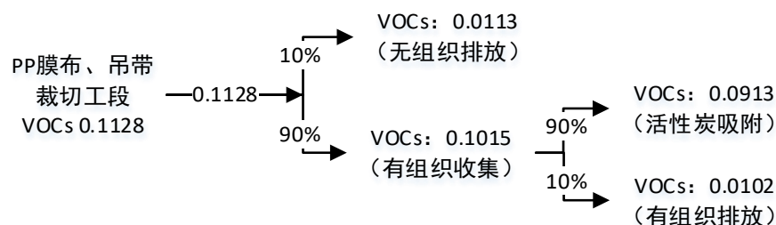
图 2-2 本项目 VOCs 平衡图 (t/a)
