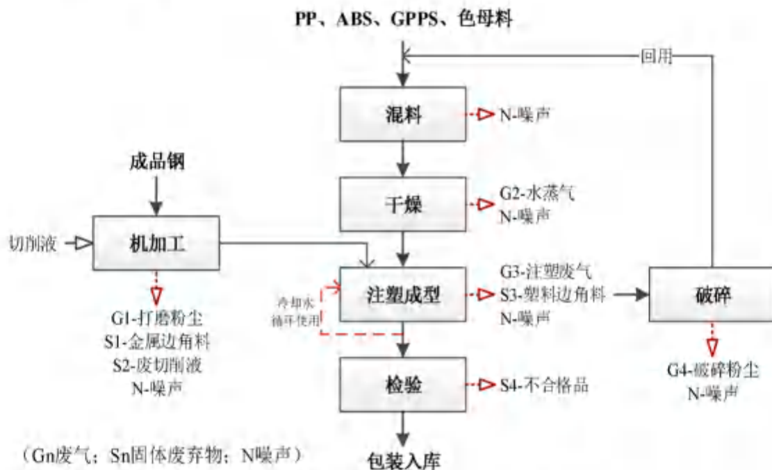
图 2-2 塑料制品生产和模具加工工艺流程图
