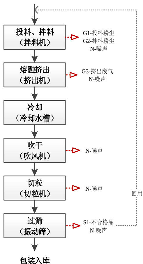
图 2-2 改性塑料粒子工艺流程图
