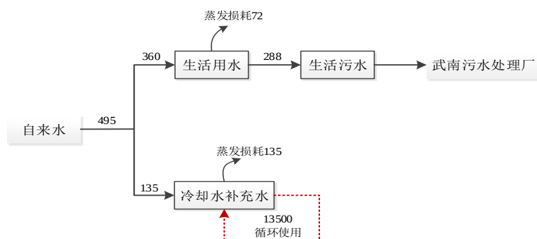
图 2-1 验收项目水平衡图 (t/a)
