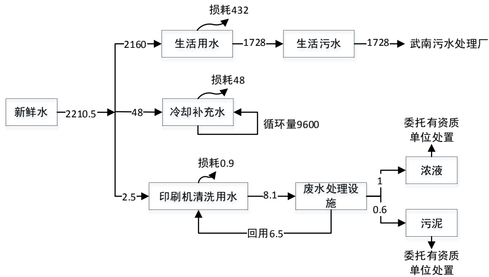
图 2-1 验收项目水平衡图 (t/a)
