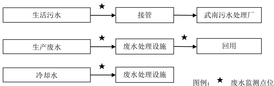
图 3-1 污水接管及监测点位图
