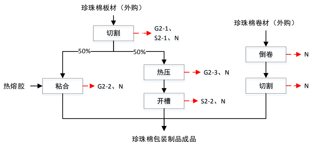
图 2-3 珍珠棉包装制品工艺流程图
