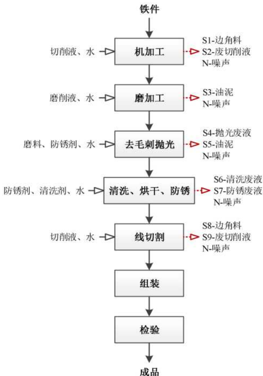
图 2-3 液压泵及配件生产工艺流程图
