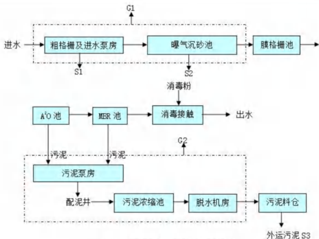
图 4-1 滨湖污水处理厂工艺流程图
