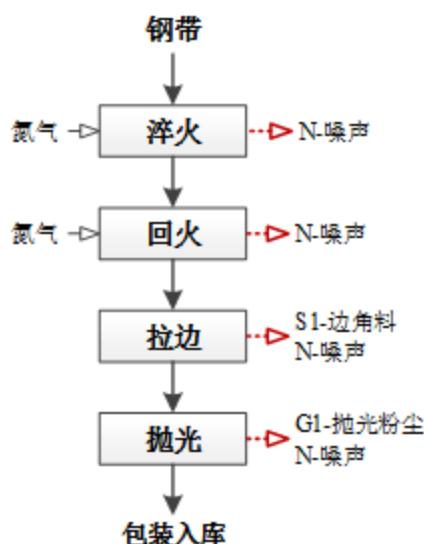
图 2-3 弹簧钢加工工艺流程图
