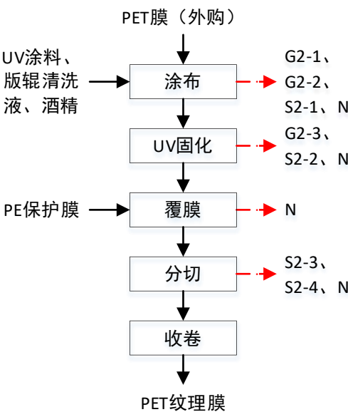
图 2-3 PET 纹理膜生产工艺流程图 (注：Gn：废气污染物；Sn：固体废弃物；N：噪声)
