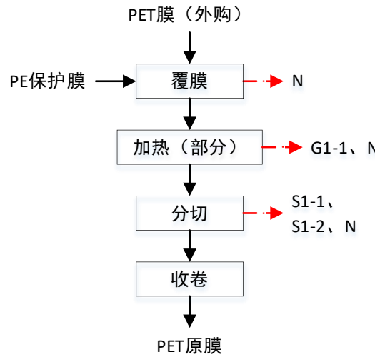
图 2-2 PET 原膜生产工艺流程图 （注：Gn：废气污染物；Sn：固体废弃物；N：噪声）
