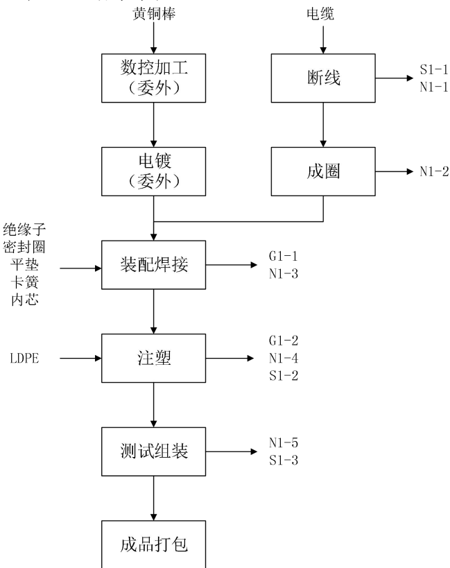
图 2-2 电缆组件生产工艺流程图
