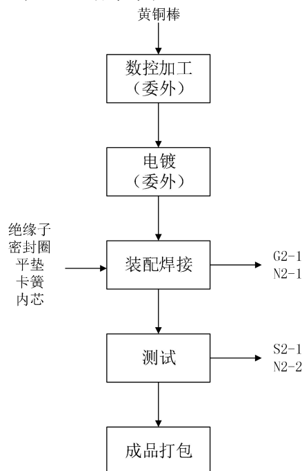
图 2-3 同轴射频连接器生产工艺流程图
