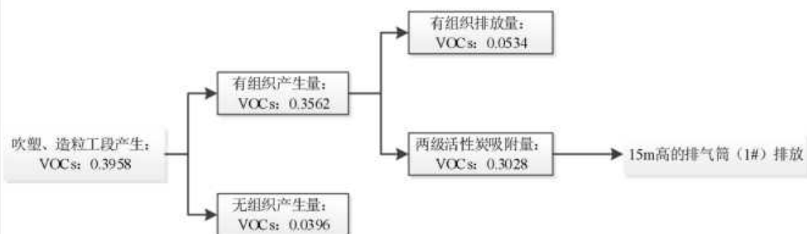
图 2-2VOCs 平衡图 (t/a)
