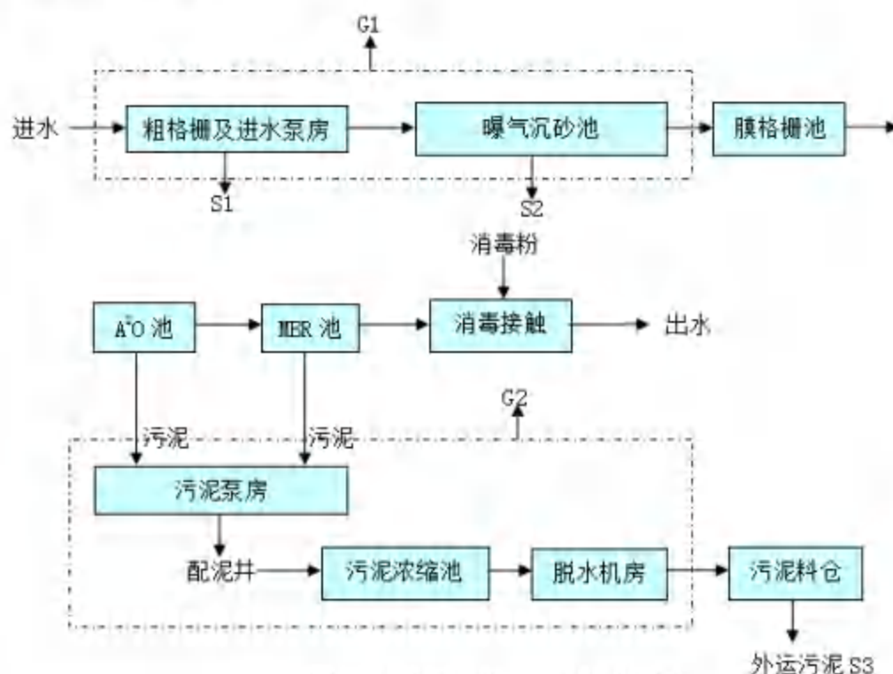
图 4-2 滨湖污水处理厂工艺流程图
