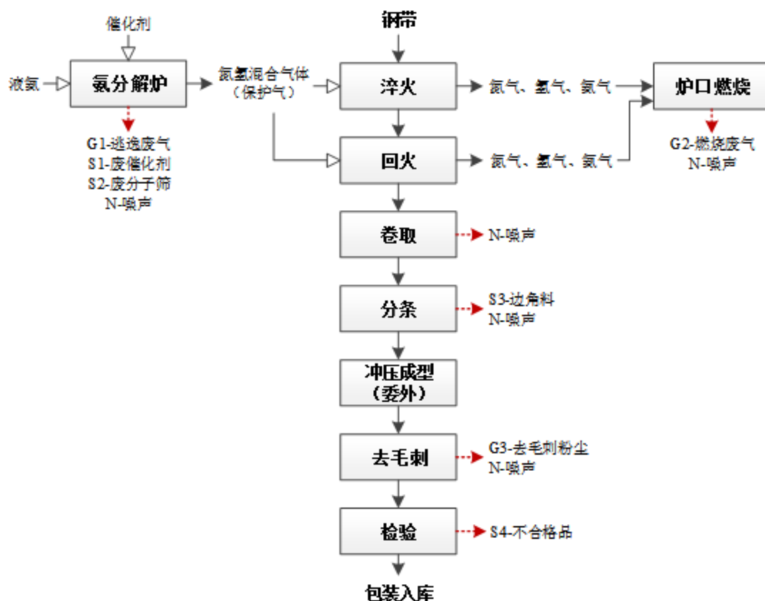
图 2-2 精密织机配件生产工艺流程图
