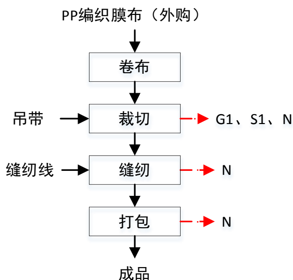
图 2-2 集装袋工艺流程图
