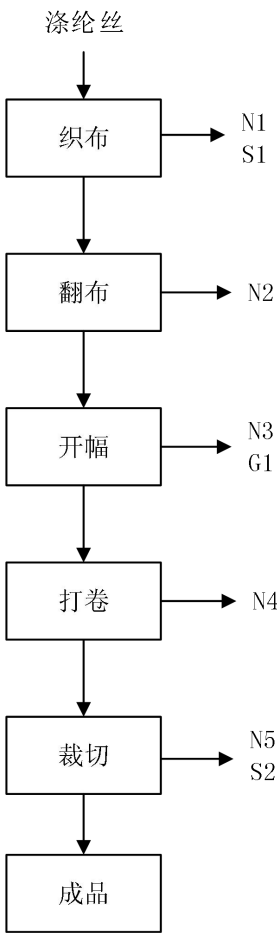
图 2-2 涤纶网布生产工艺流程图 (注: Gn: 废气污染物; Sn: 固体废弃物; N: 噪声)
